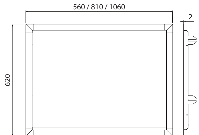
Telaio a filo per armadietto Slim Frame (smooth version)
