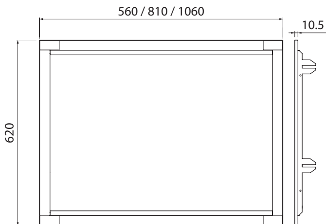
Telaio rialzato per armadietto Slim Frame (thick version)
